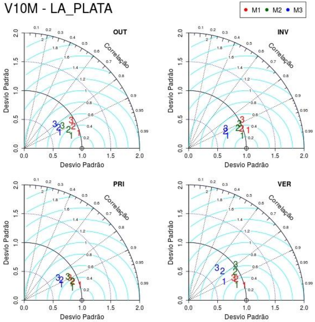
Figura H4. Idem à Figura H1 para a região de La Plata.
