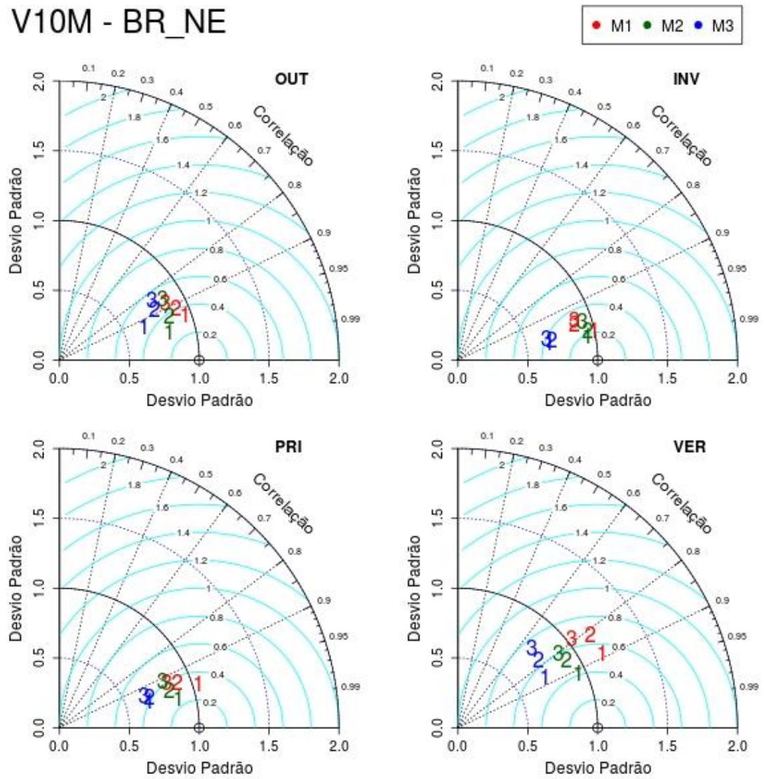
Figura H2. Idem à Figura H1 para a região Nordeste.
