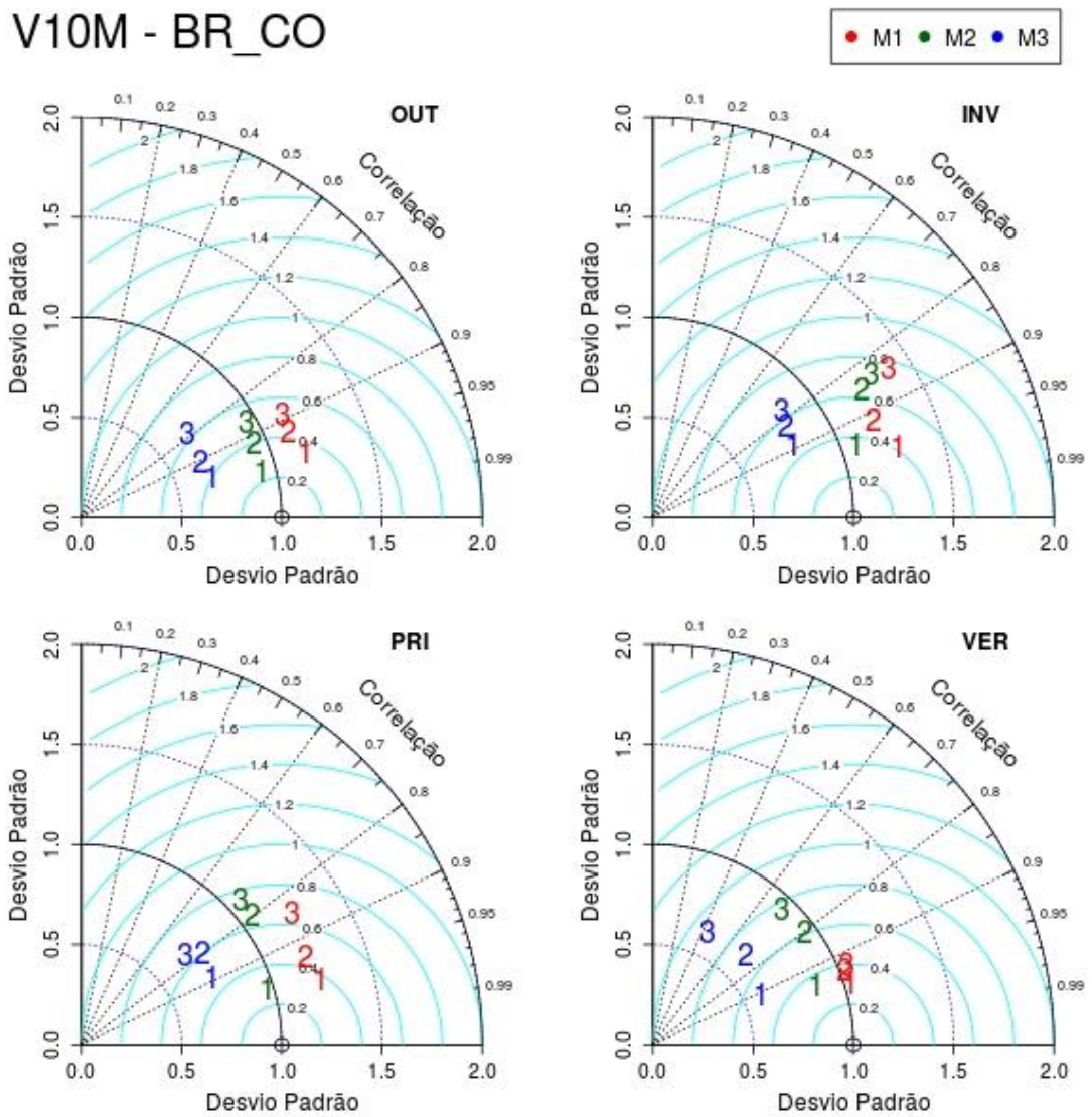
Figura H1. Diagrama de Taylor para a região Centro-Oeste para a) outono, b) inverno e c) primavera de 2016 e d) verão de 2016/17.
