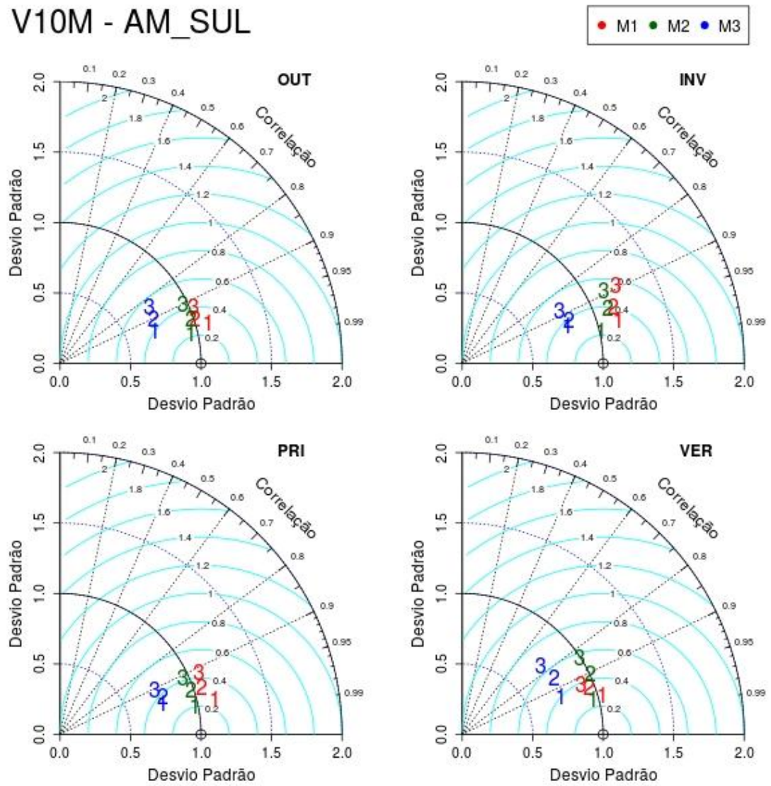
Figura H5 Idem à Figura H1 para a região América do Sul.
