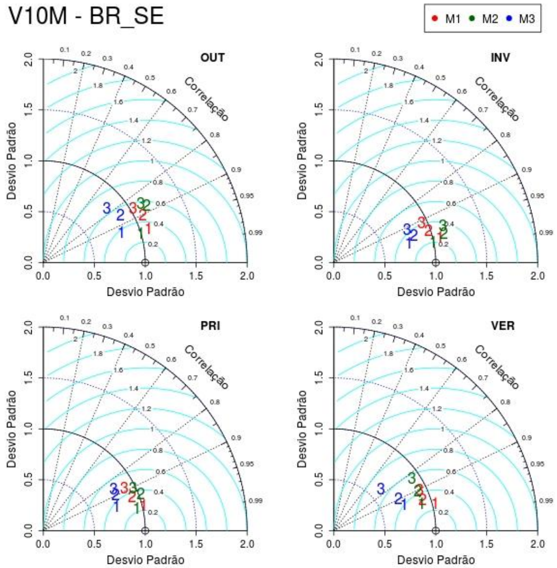
Figura H3. Idem à Figura H1 para a região Sudeste.
