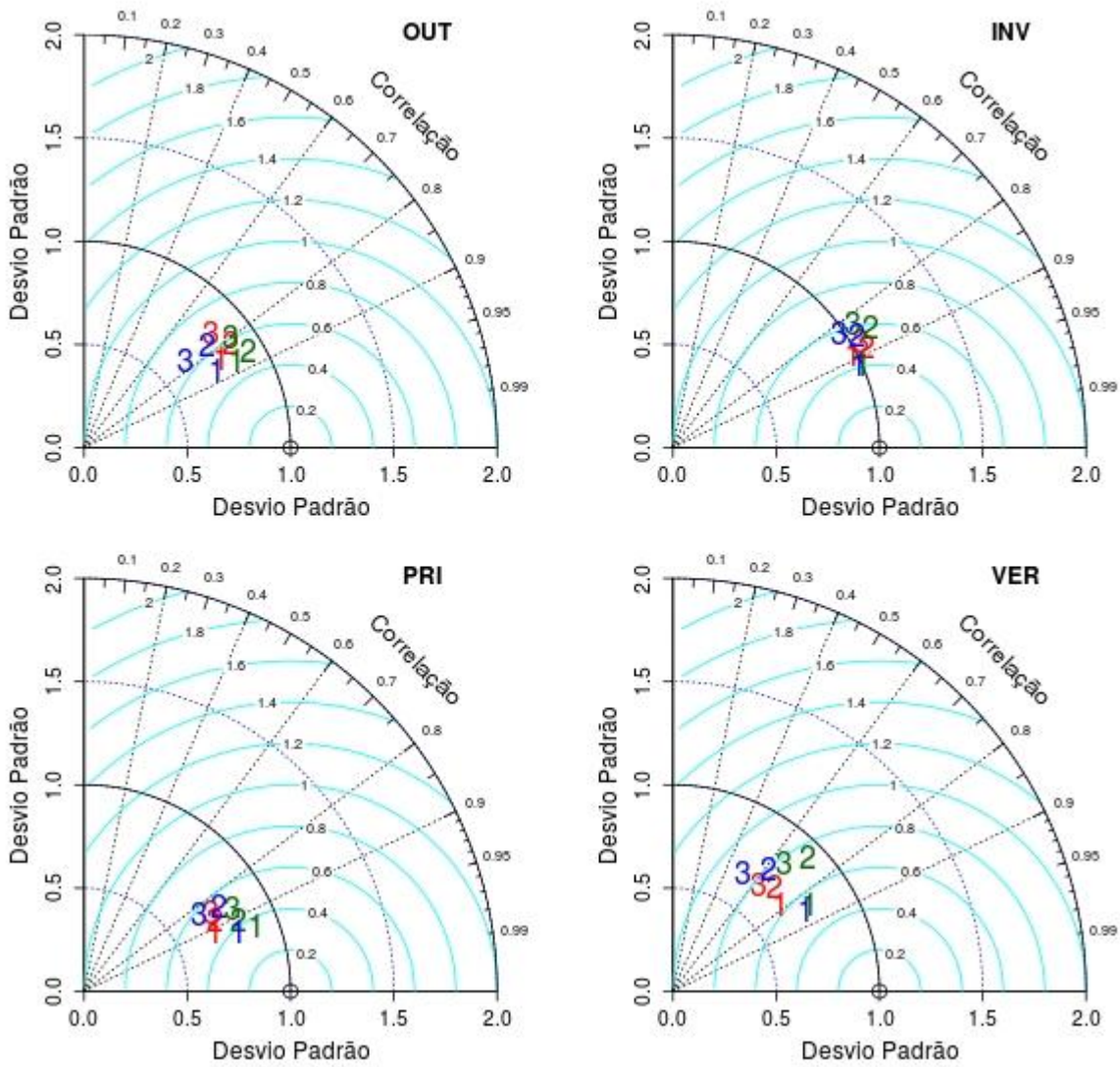
Figura D4. Diagrama de Taylor para a região da bacia de La Plata, a) outono, b) inverno e c) primavera de 2016 e d) verão de 2016/17.
