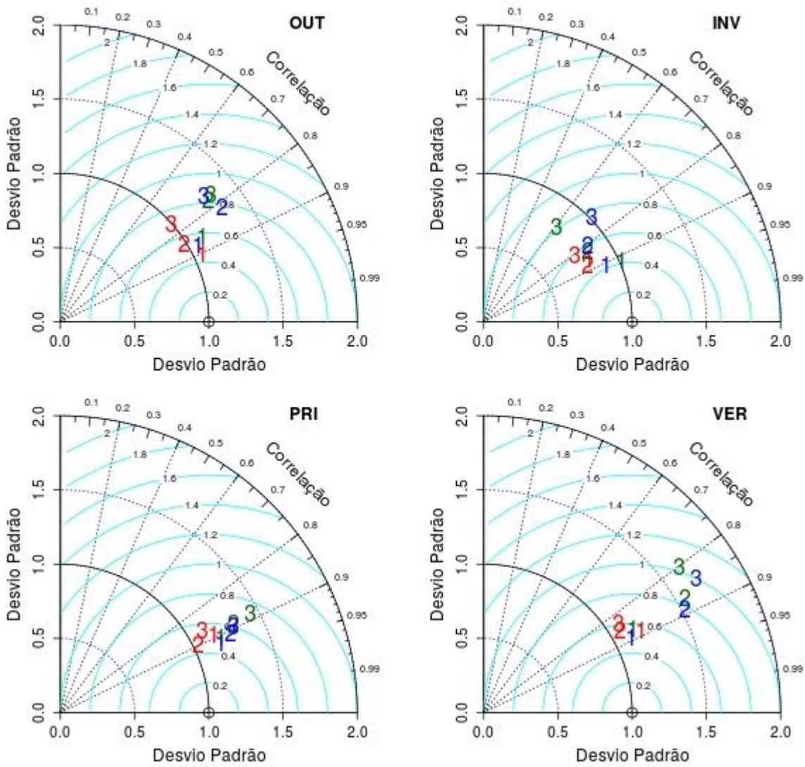
Figura D3. Diagrama de Taylor para a região Sudeste, a) outono, b) inverno e c) primavera de 2016 e d) verão de 2016/17.
