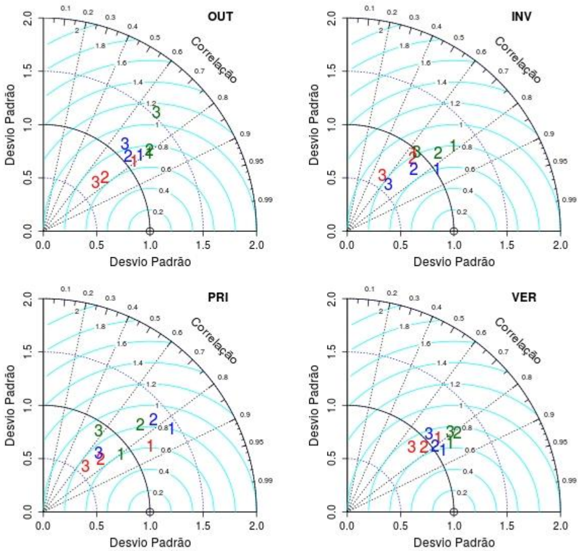
Figura D2 Diagrama de Taylor para a região Nordeste, a) outono, b) inverno e c) primavera de 2016 e d) verão de 2016/17.
