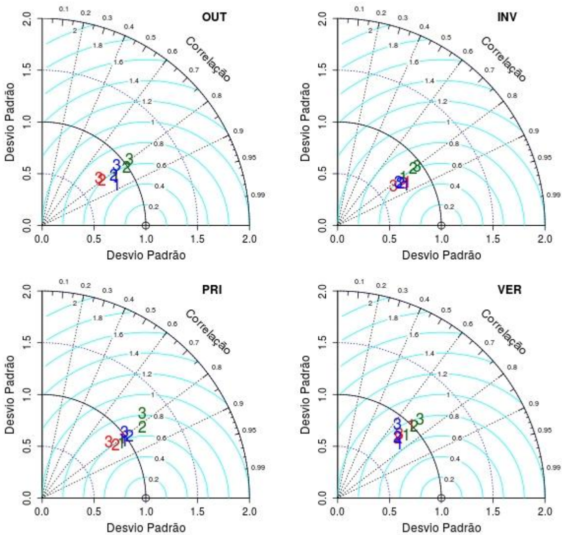
Figura D5. Diagrama de Taylor para a região da América do Sul, a) outono, b) inverno e c) primavera de 2016 e d) verão de 2016/17.
