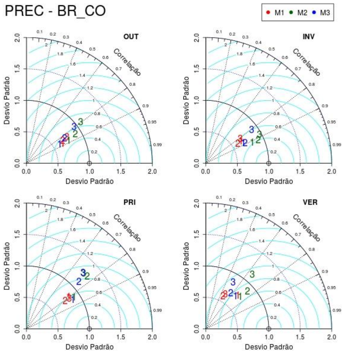
Figura D1. Diagrama de Taylor para a região Centro-Oeste, a) outono, b) inverno e c) primavera de 2016 e d) verão de 2016/17.
